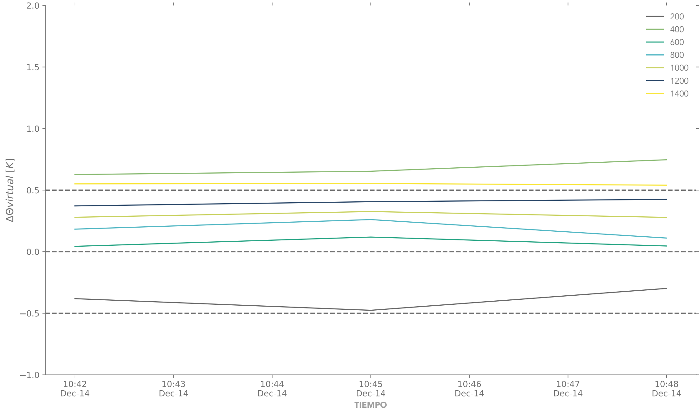
ÍNDICE DE ESTABILIDAD ATMOSFÉRICA \Delta\Theta VIRTUAL A DIFERENTES NIVELES DE ALTURA
